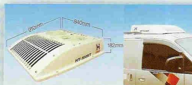
Waga ~ 18kg Skraplacz dachowy
